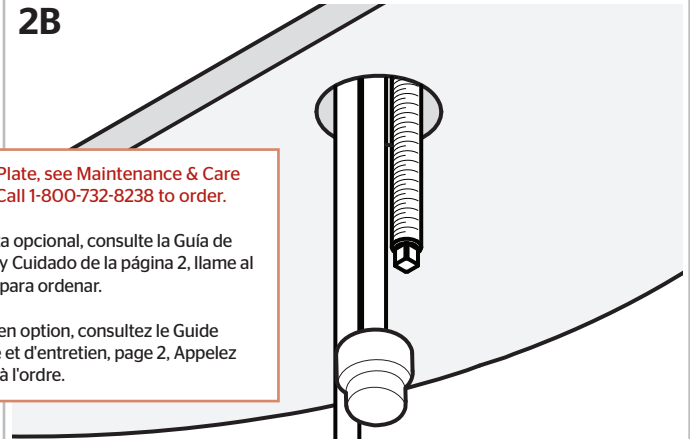
Optional Deck Plate (not included) Placa de cubierta opcional (no incluido). Plaque de pont en option (non inclus).
